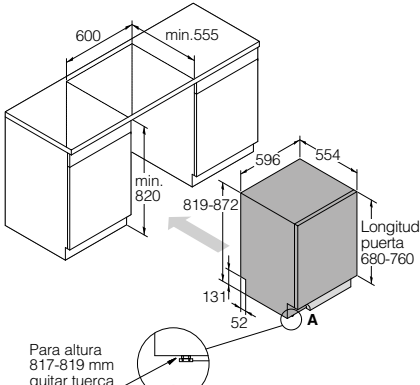
Dimensiones de instalación
