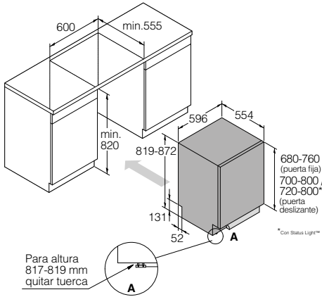
Dimensiones de instalación
