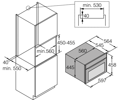
Instalación en columna
