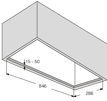
Dimensiones del hueco
