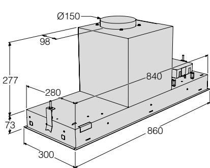
Dimensiones del aparato
