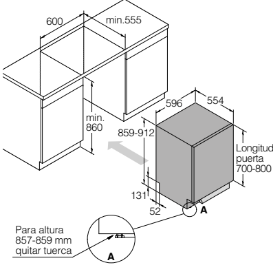
Dimensiones de instalación
