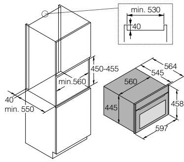
Instalación en columna
