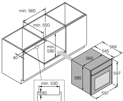
Instalación bajo encimera
