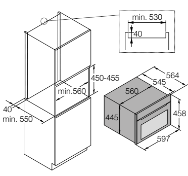
Instalación en columna
