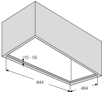
Dimensiones del hueco
