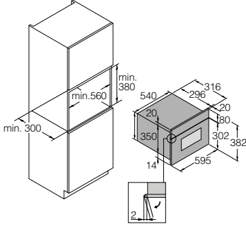
Instalación en columna
