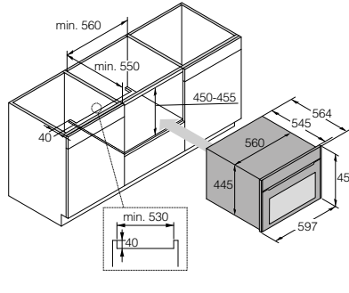
Instalación bajo encimera
