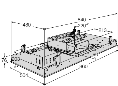
Dimensiones del aparato
