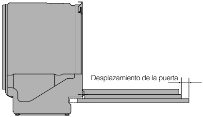
Instalación con puerta deslizante XL/XXL
