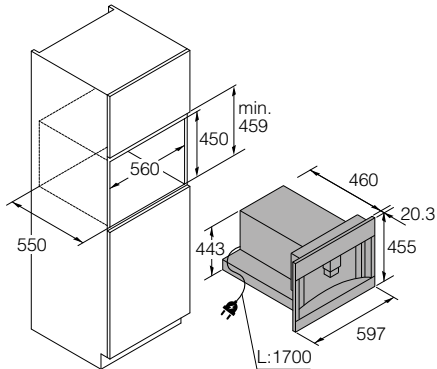
Dimensiones del electrodoméstico y del nicho de instalación
