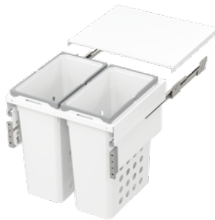
Ancho de mueble 600 mm 2 cubos, 88L (2x44L)
